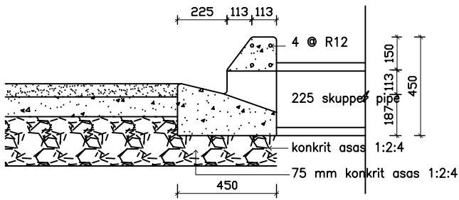
KERATAN
