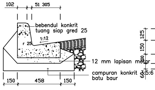
(KERATAN TIPIKAL BEBENDUL JALAN)
